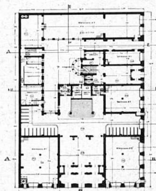
ПЛАНЪ I этажа
